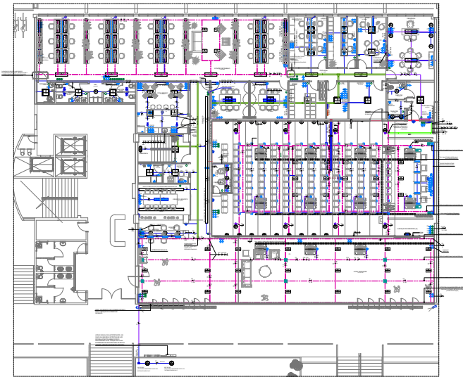
10 PLANTA BAJO TERREO
