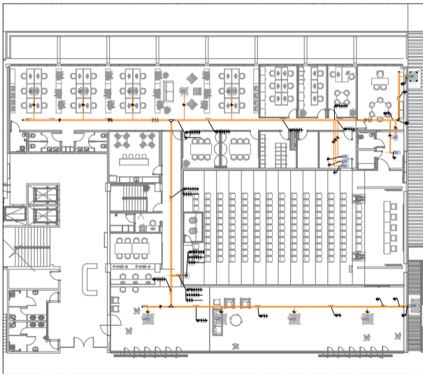
11- PLANTA BAIXA - TERREO NOVAS INSTALAÇÕES escala: 1:50
