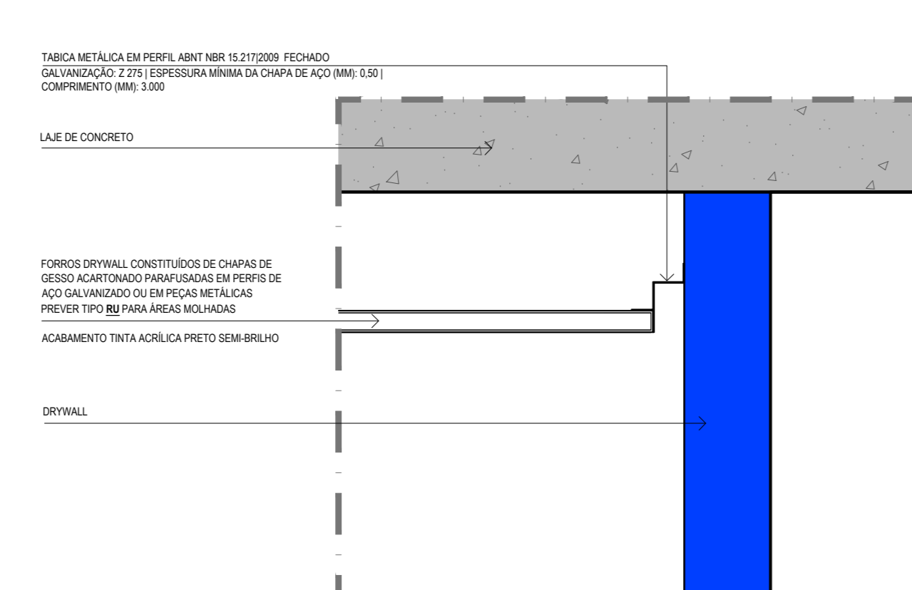
DET.-02 | TABICA METÁLICA OBRIGATORIA EM TODOS OS AMBIENTES COM FORRO DE GESSO ESCALA 1:5
