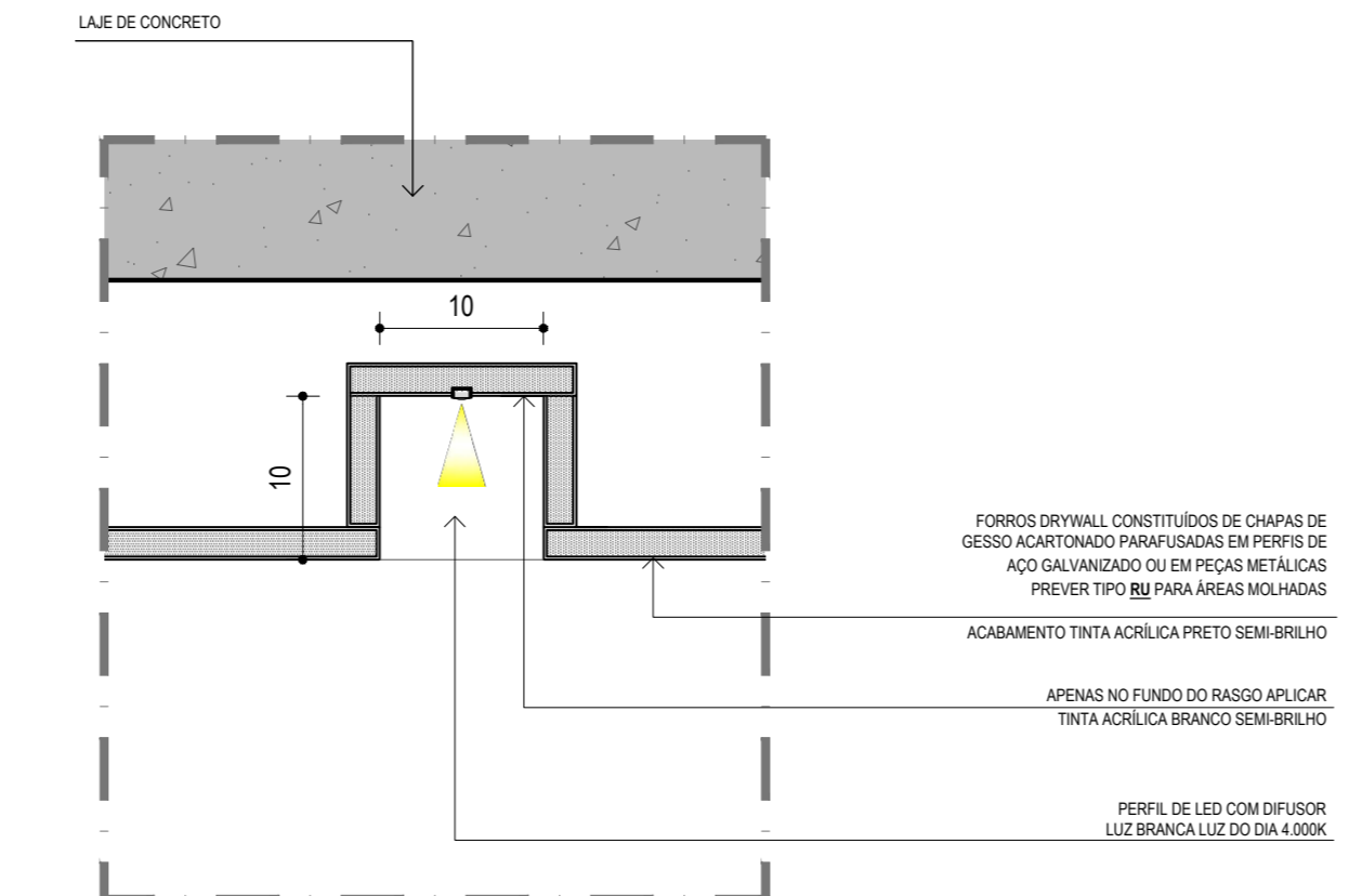
DET.-03 | RASGO REBAIXO CIRCULAÇÃO ESCALA 1:5
