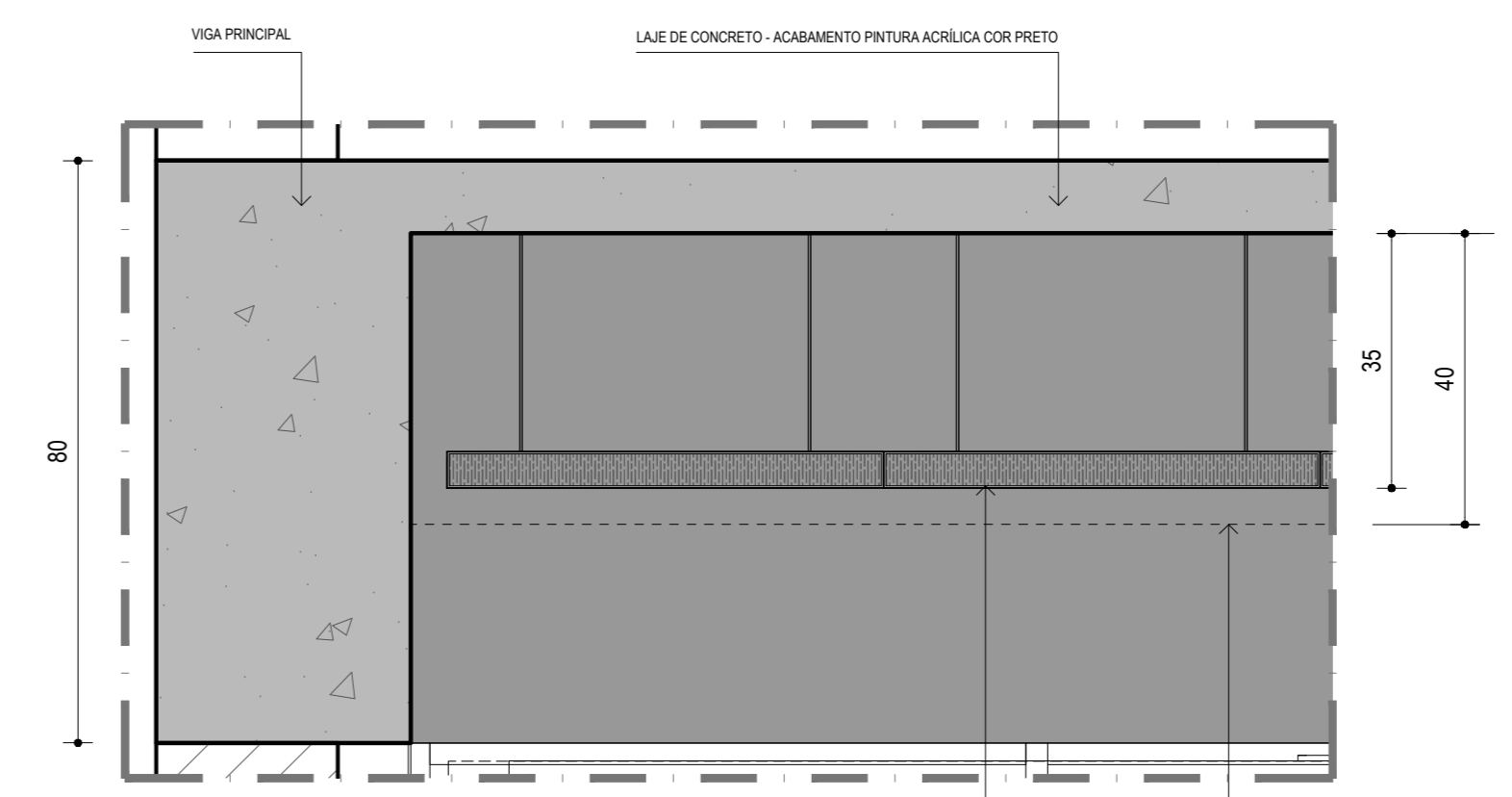
DET.-04 | NUVEIS ACÚSTICAS EM LÂ DE PET ESCALA 1:10
