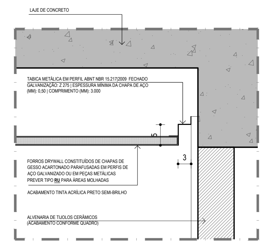
DET.-01 | TABICA METÁLICA OBRIGATORIA EM TODOS OS AMBIENTES COM FORRO DE GESSO ESCALA 1:5
