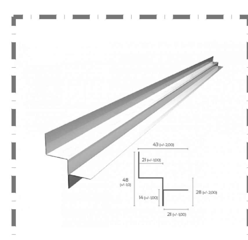
IMAGEM TABICAS METÁLICAS ESCALA 1:5
